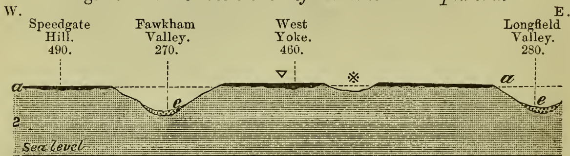
Fig. 1.— Transverse section of the West-Yoke plateau.
